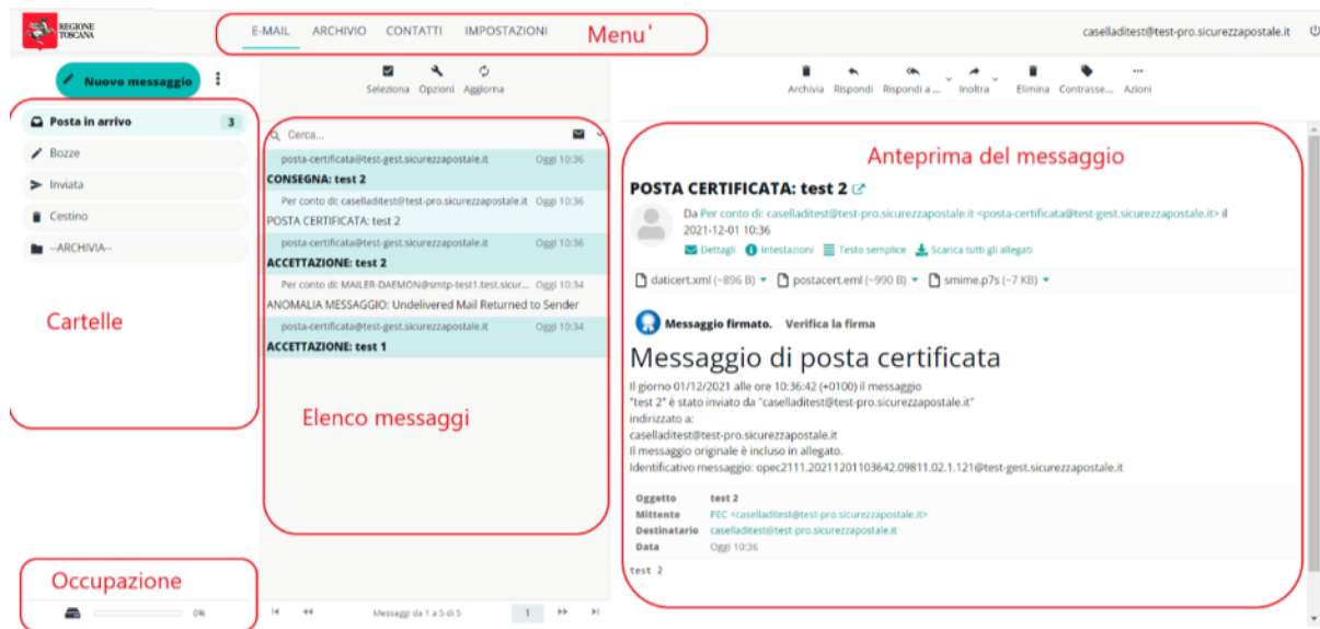
Figura 2 – Schermata principale
